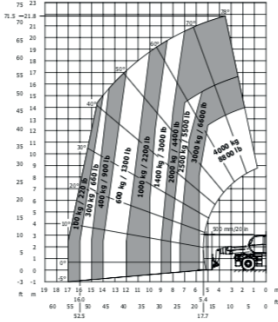
Frontale su pneumatici con forche EN 1459
