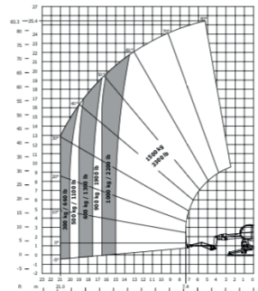
Rotazione su stabilizzatori estesi con braccetto 1500 kg EN 1459
