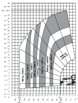
Rotazione su stabilizzatori estesi con argano 5000 kg EN 1459
