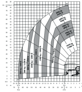
Rotazione su stabilizzatori estesi con forche EN 1459
