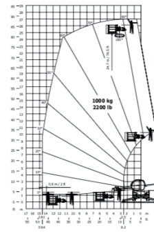
Rotazione su stabilizzatori estesi con cestello 1000 kg EN 280
